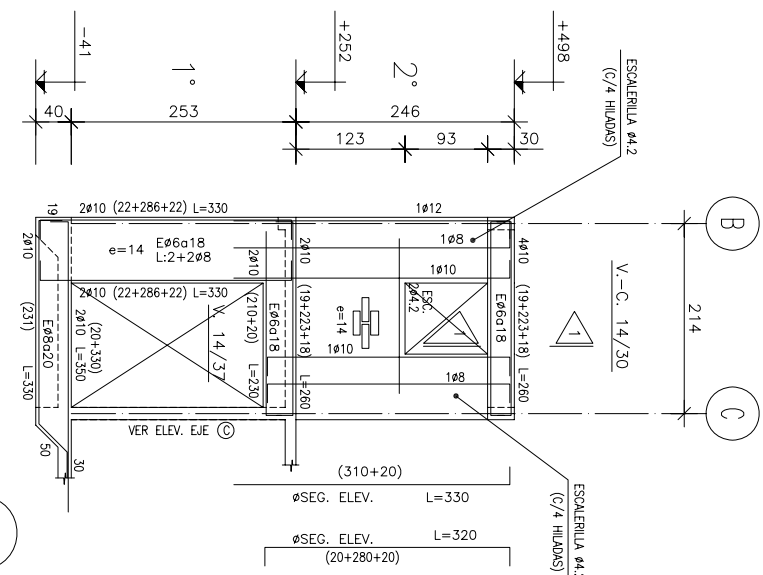
ELEVACION EJE 2
