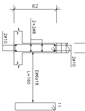
SECCION 5-5
