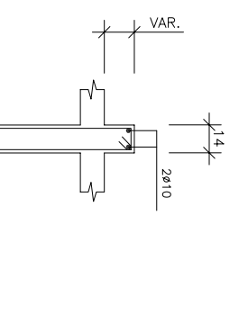
SECCION 7-7
